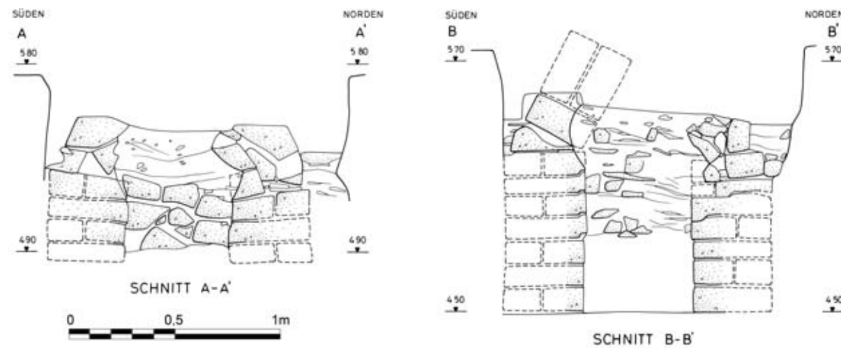
Abb. 242 F/I-n/21-Grab 6, Schnitte A-A' und B-B'
