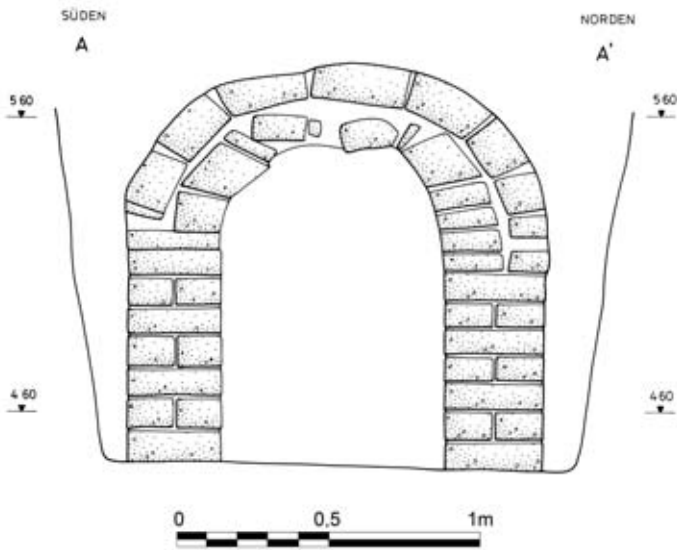
Abb. 247 F/I-n/21-Grab 10, Schnitt A–A'
