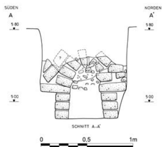
Abb. 256 F/I-o/21-Grab 2, Schnitt A-A'
