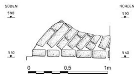
Abb. 252 F/I-n/22-Grab 1, Ansicht des Gewölbes von Osten
