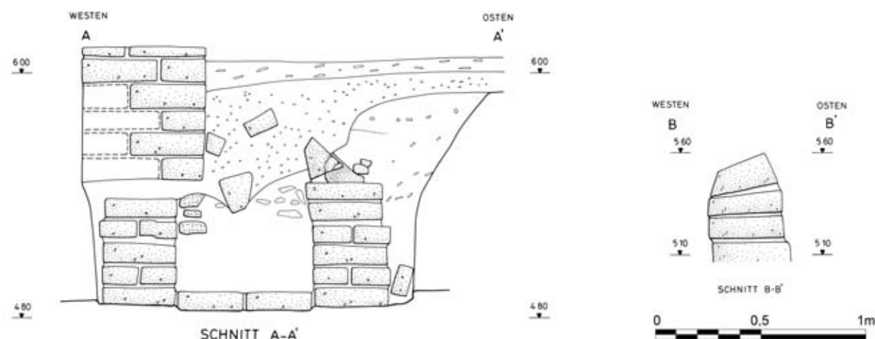
Abb. 271 F/I-p/21-Grav 2, Schnitte A-A' und B-B'
