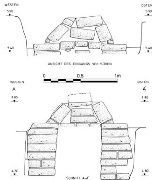
Abb. 251 F/I-n/22-Grab 1, Ansicht des Eingangs und Schnitt A-A'
