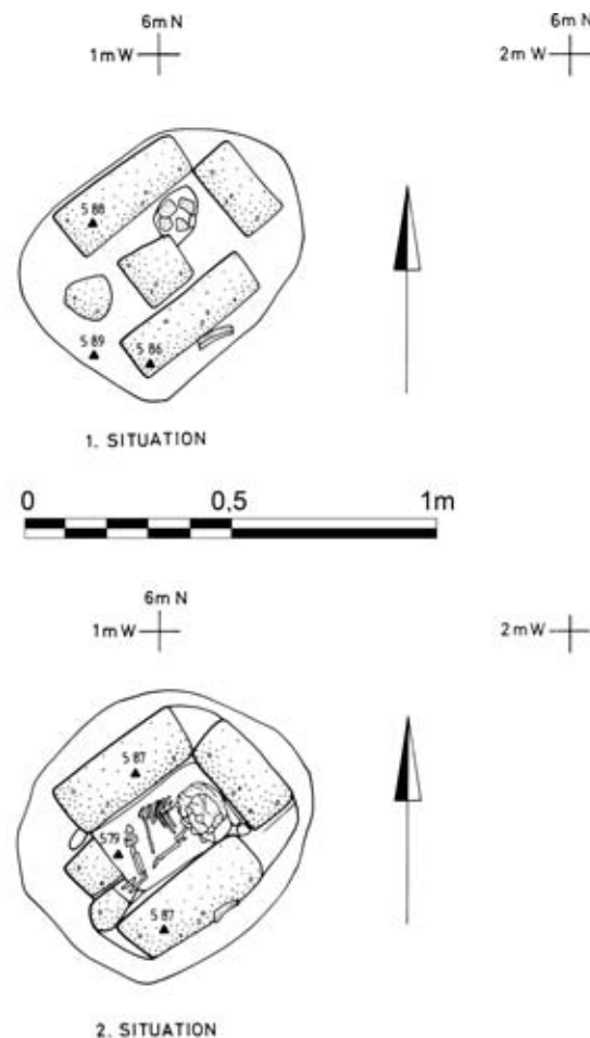
Abb. 243 F/I-n/21-Grab 9, 1. und 2. Situation
