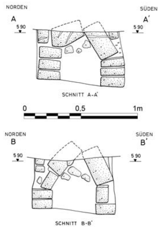
Abb. 238 F/I-n/21-Grab 1, Schnitte A-A' und B-B'
