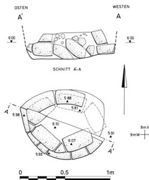
Abb. 234 F/I-n/20-Grab 11 , 1. Situation und Schnitt A–A'
