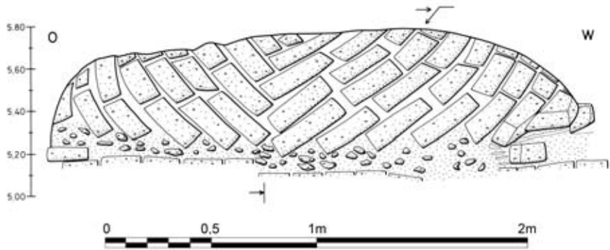
Abb. 246 F/I-n/21-Grab 10, Ansicht des Gewölbes von Norden
