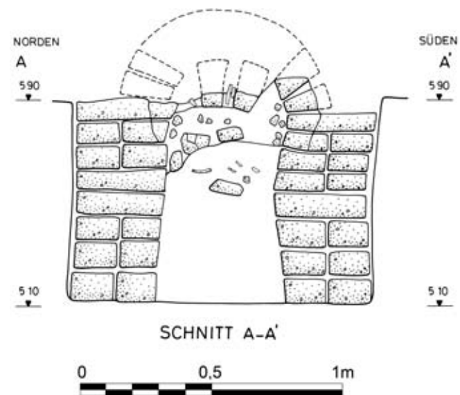
Abb. 263 F/I-o/21-Grab 7, Schnitt A–A'
